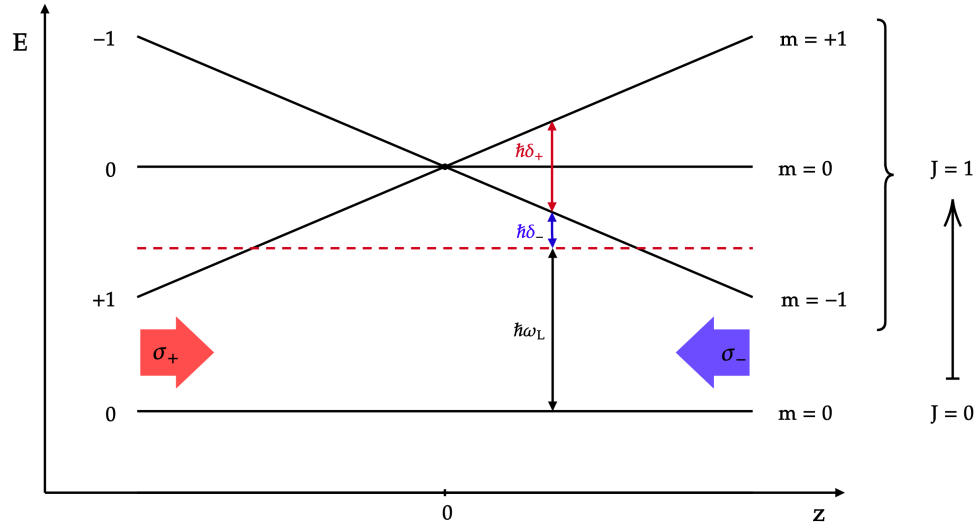
Slika 2.4: Ilustracija cijepanja energetskih nivoa za dvorazinski atom u gradijentu polja anti Helmholtzovih zavojnica.
