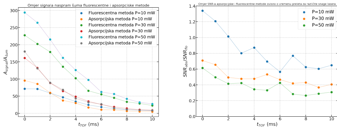
Slika 5.7: SNR fluorescentne i apсорpcijske metode oslikavanja u ovisnosti o vremenu proleta za različite snage lasera za hlađenje (lijevo). Omjer SNR -a apсорpcijske i fluorescentne metode ovisno o vremenu proleta za različite snage lasera za hlađenje.
