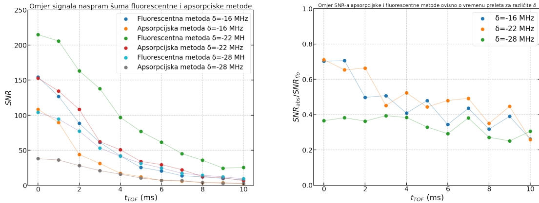
Slika 5.6: SNR fluorescentne i apsorpcijske metode oslikavanja u ovisnosti o vremenu proleta za različite pomake frekvencije lasera za hlađenje (lijevo). Omjer SNR -a apсорpcijske i fluorescentne metode ovisno o vremenu proleta za različite pomake frekvencije lasera za hlađenje.
