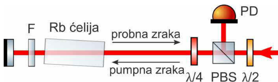
Slika 3.5: Shematski prikaz postava za saturacijsku apsorpcijsku spektroskopiju. Oznake: PBS-polarizacijski djelitelj zrake; F-filter; \lambda/4 , \lambda/2 - polarizacijske pločice; PD-fotodioda.
