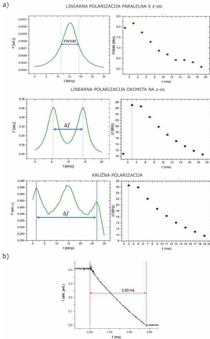
Slika 3.11: a) Sila zračenja na hladni atomski oblak ^{87}\text{Rb} u ovisnosti o frekvenciji za različite polarizacije probne zrake. (lijevo). Širina na pola visine (FWHM) i razmak između rascijepljenih linija za odgovarajuće polarizacije probne zrake u različitim vremenima nakon gašenja struje kroz anti-Helmholtz zavojnice (desno). b) Vremenska relaksacija struja kroz anti-Helmholtz zavojnice.
